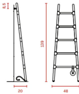
SCALETTA 140
