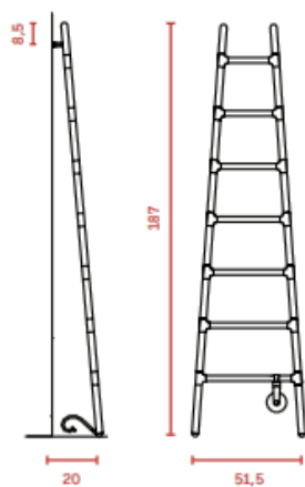
SCALETTA 185
